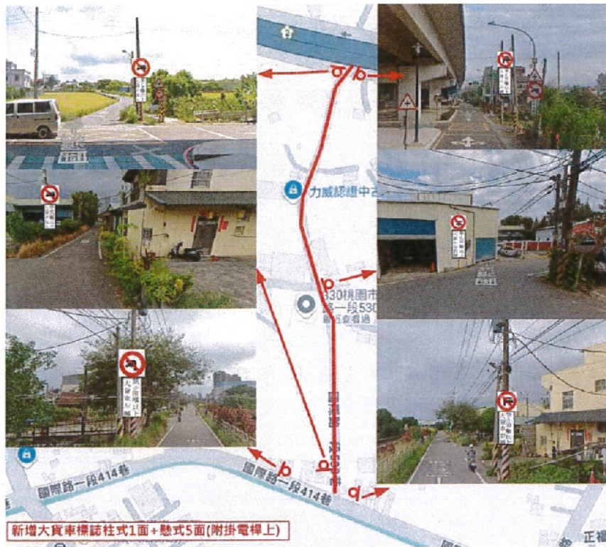
圖 1 禁行路線圖
