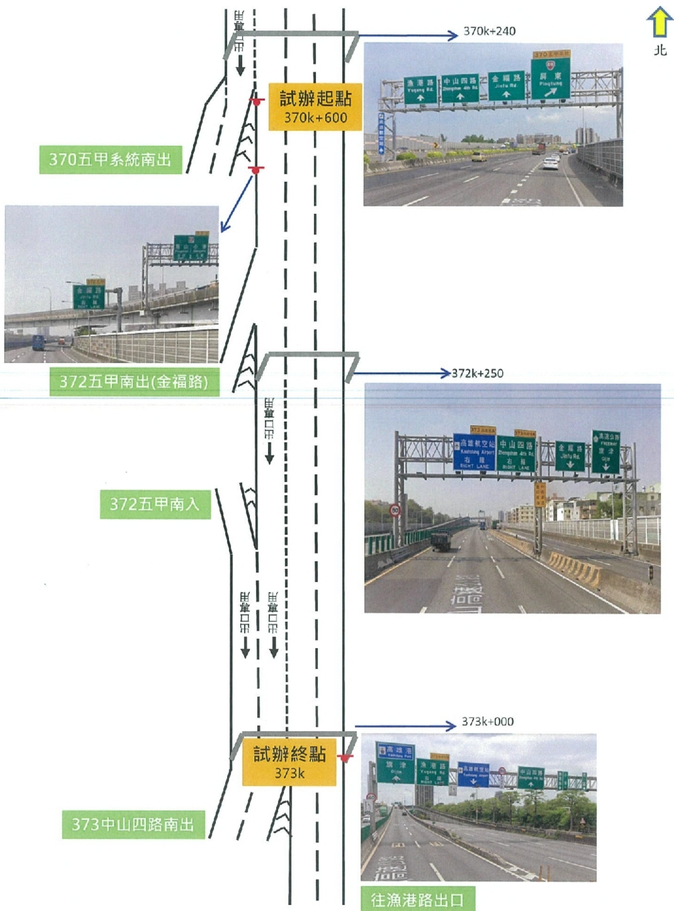
國1南向五甲系統出口後至高雄端試辦「車道不限車種通行」措施示意圖
